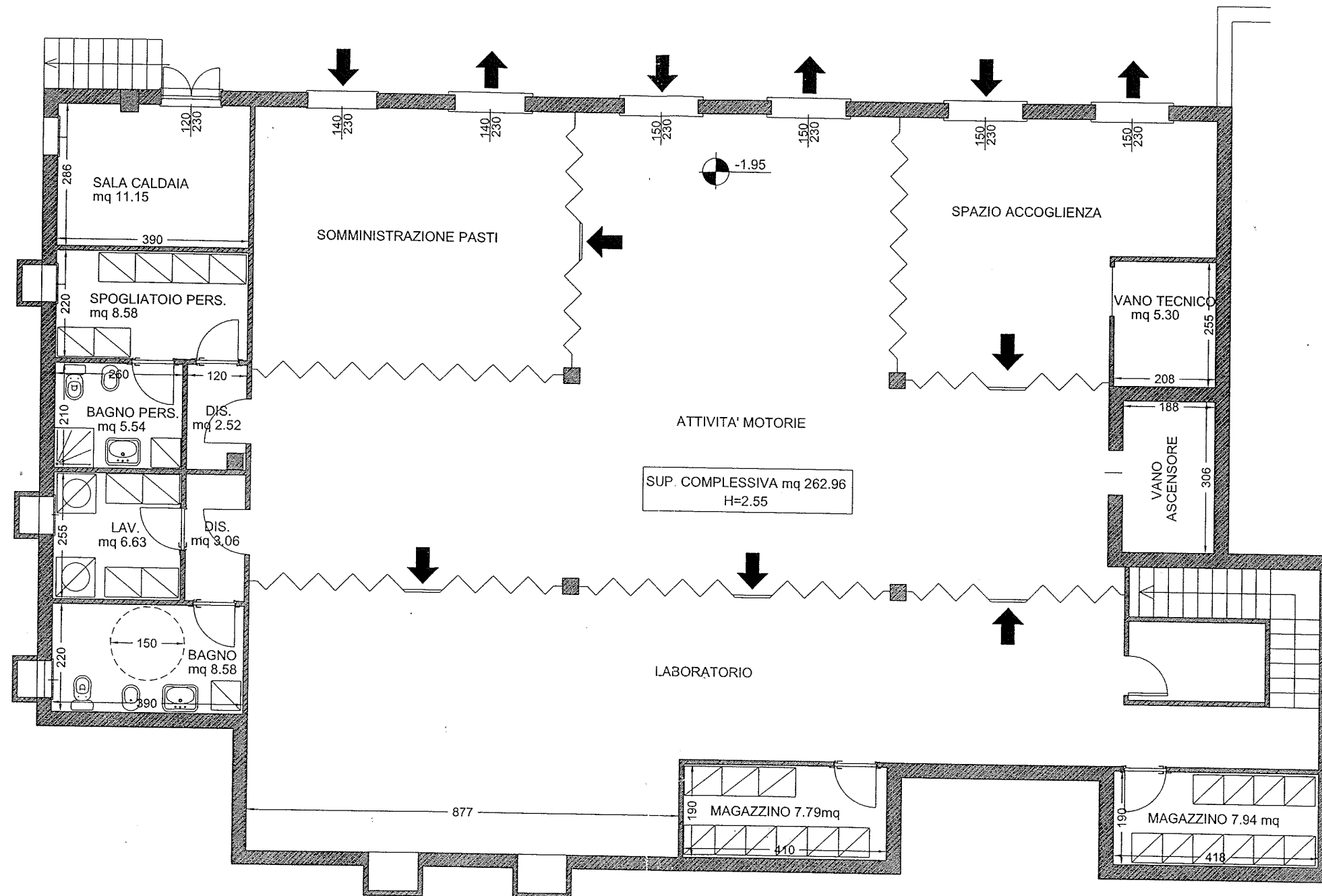
PIANTA SEMINTERRATO SCALA 1:100
