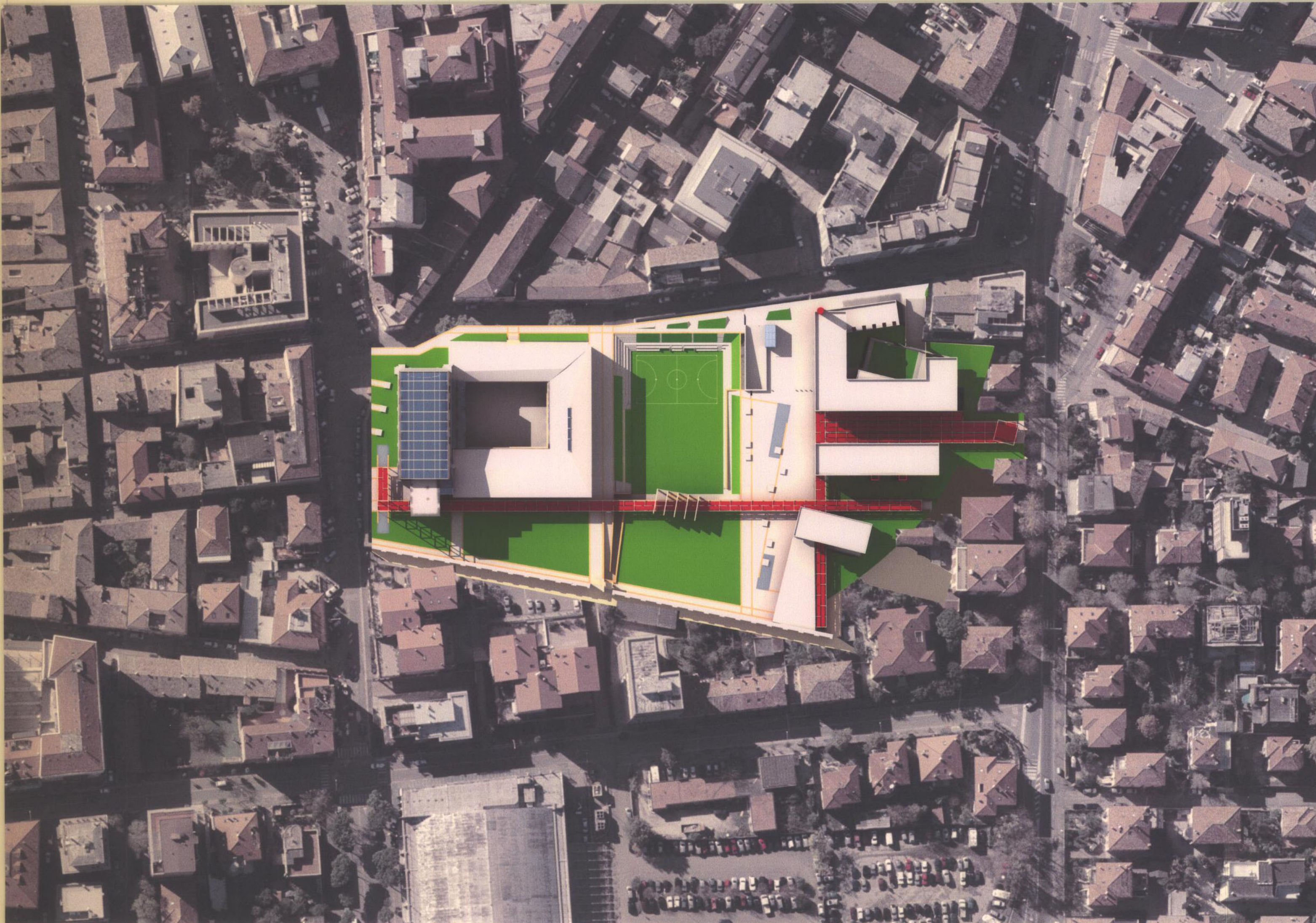
PLANIVOLUMETRICO RAPP. 1:1000
