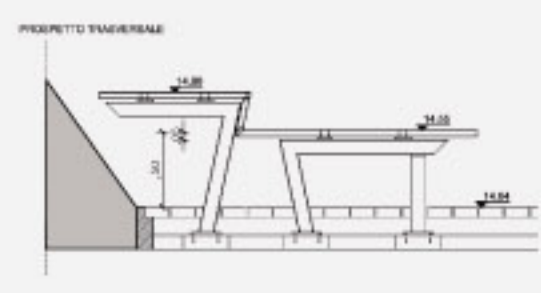
PANCHINA - TIPOLOGIA A scala 1:20
