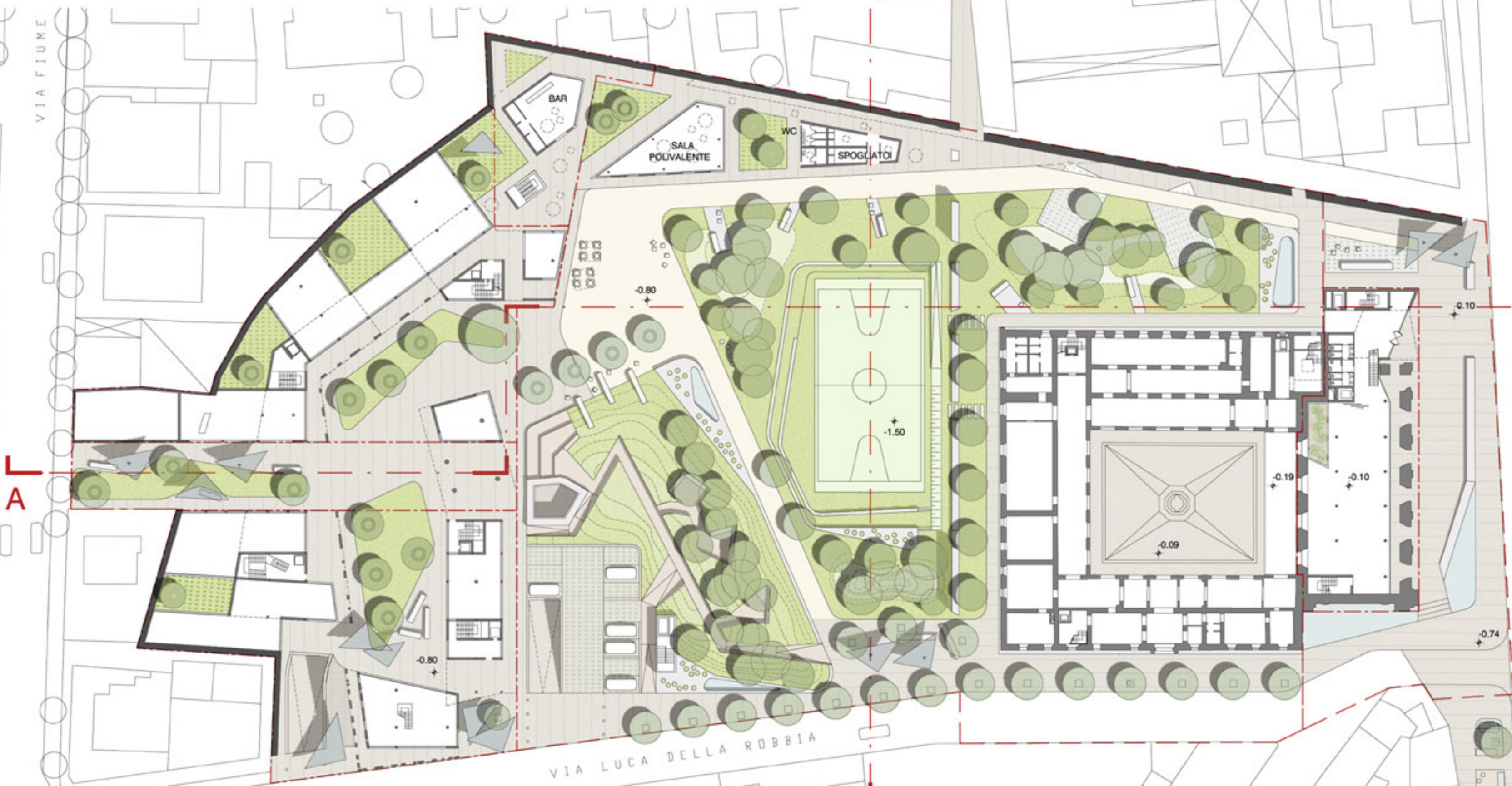
PIANTA PIANO TERRA PARCO PUBBLICO -0.80 1:500
