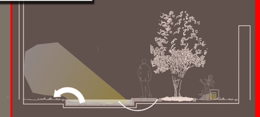
sezione c-c
