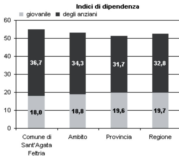
Grafico 1.2 Indici di vecchiaia e di dipendenza al 31/12/2000
